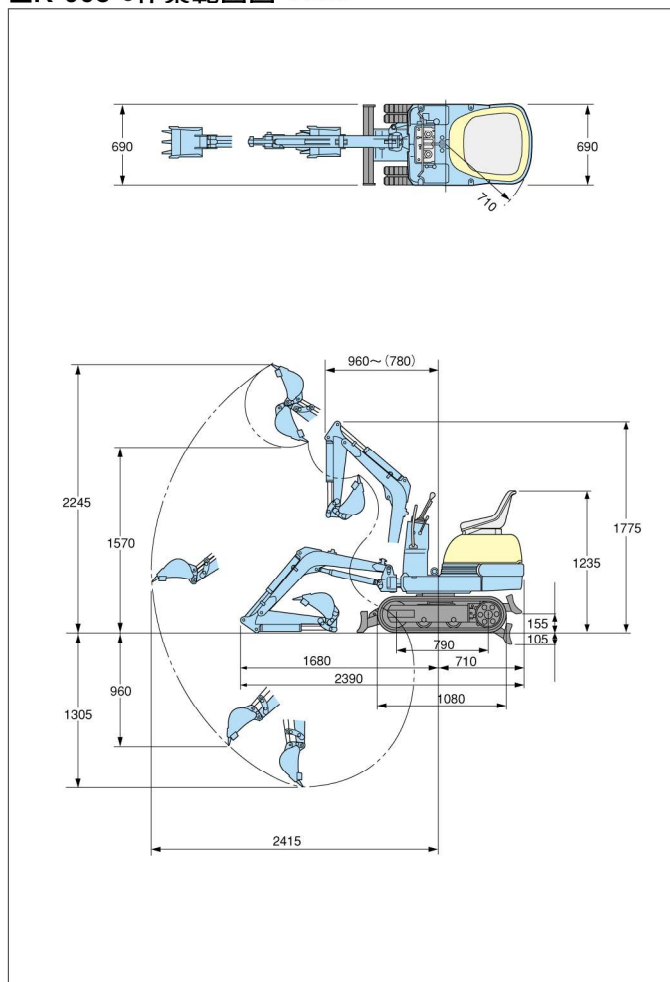
■K-005-3作業範囲図 単位:mm
