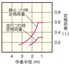
RX-205 CR 定格荷重 (標準アーム、0.06m 3 バケット付)
