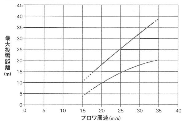
【最大投雪距離】
