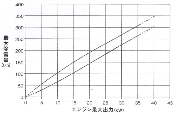
【最大除雪能力】
