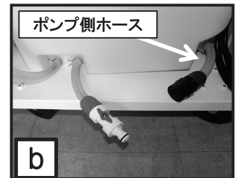
排水
